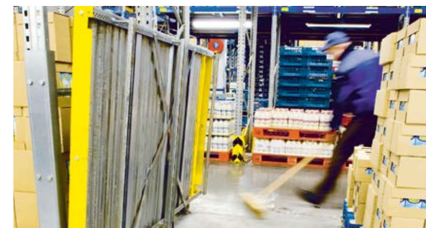
Výklopné valčekové dráhy na zjednodušenie čistenia
