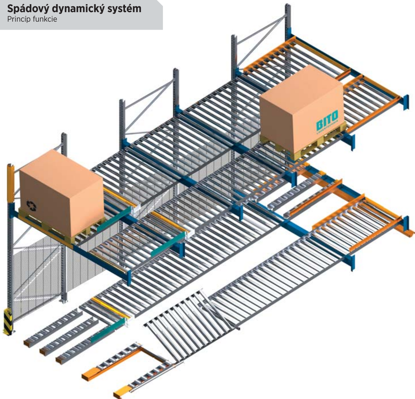
Spádový dynamický regál - FIFO princíp
