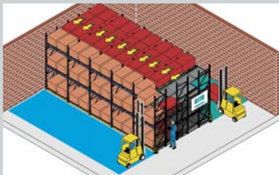
Spádový dynamický regál - FIFO princíp
