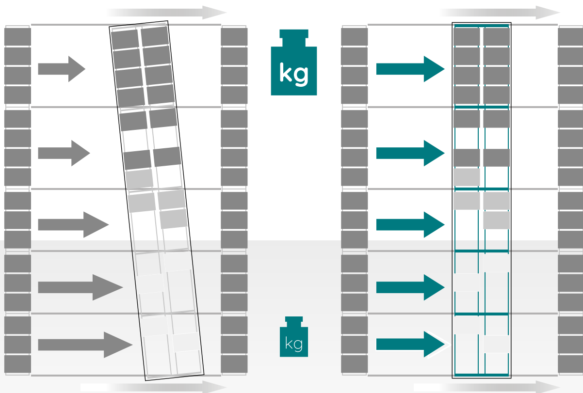
Rayonnage aux charges réparties non uniformément, sans fonction de déplacement synchronisé des bases mobiles
