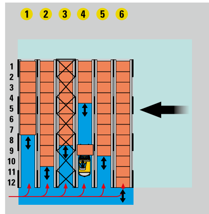
Stockage par accumulation à couloirs non traversants
