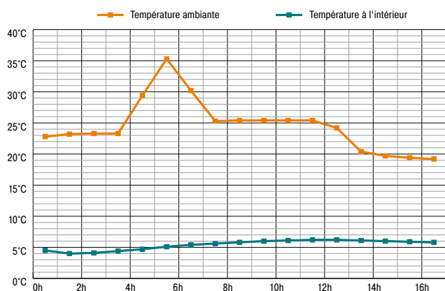
Ligne temps-température „été“ obtenue avec le set
