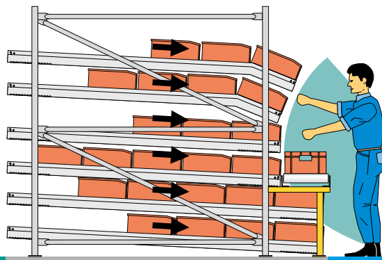
Conception ergonomique de l'avant du rayonnage
