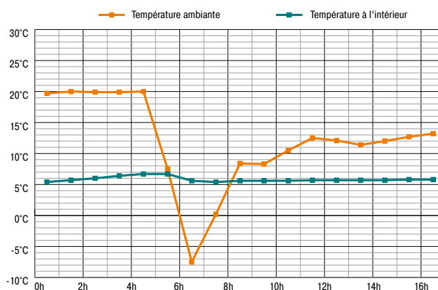
Ligne temps-température „hiver“ obtenue avec le set
