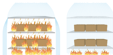
A gauche : propagation du feu avec tablettes à surface fermée A droite : propagation du feu avec tablettes grillagées perméables à l'eau
