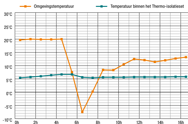
Temperatuurprofiel „winter“ van het thermo-isolatieset
