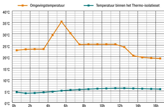
Temperatuurprofiel „zomer“ van het thermo-isolatieset
