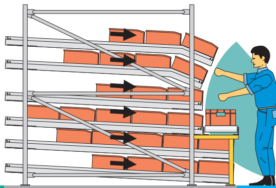
Umožňuje ergonomickú realizáciu čela regála
