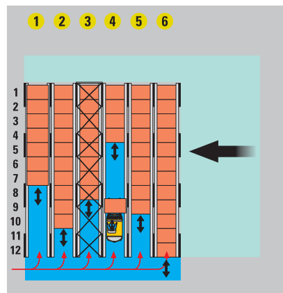
System vjazdový regál
