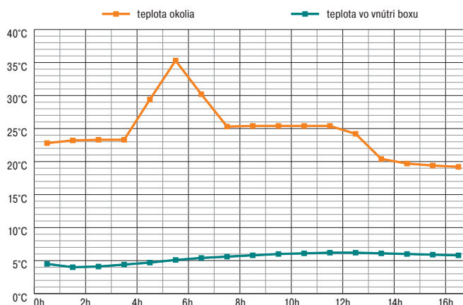
Teplotná krivka termo-izolačného setu letná
