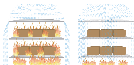
vľavo: šírenie požiaru pri uzatvorených úrovniach vpravo: šírenie požiaru pri vode priepustných úrovniach
