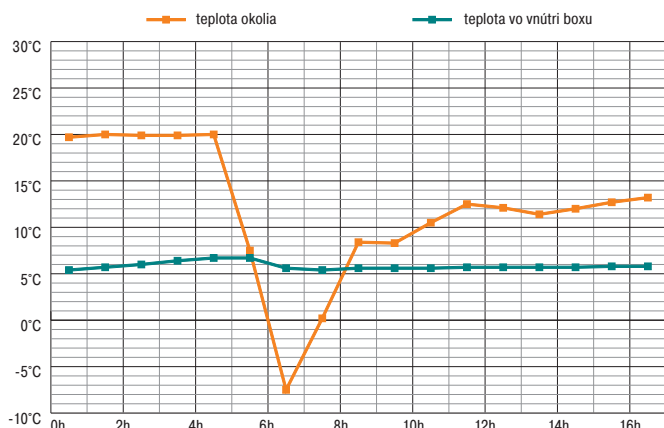
Teplotná krivka termo-izolačného setu zimná
