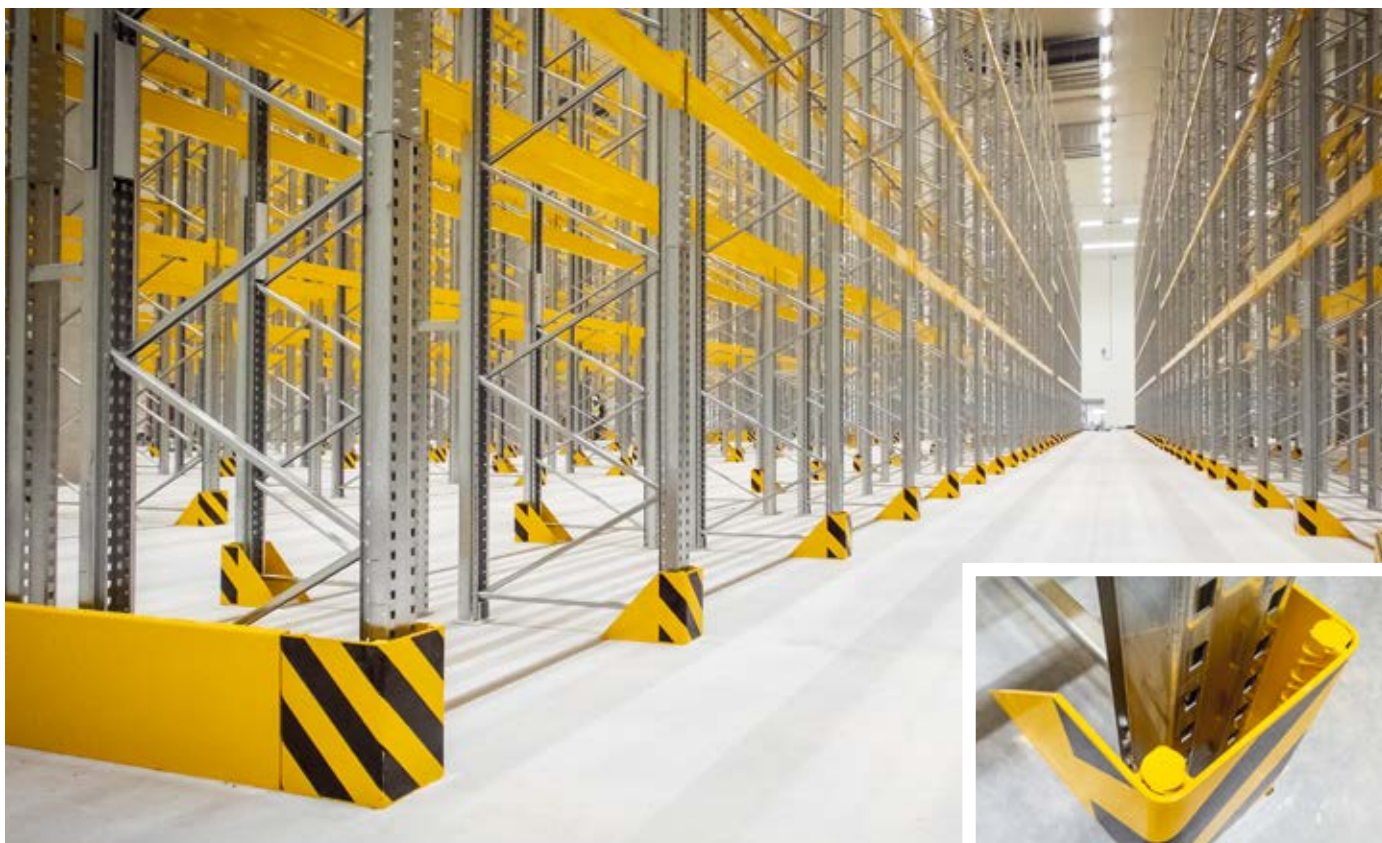
Distribučné centrum pre retail - detail obrázok mrazeného skladu, obrázok vpravo detail ochrany stojky - zákaznícke riešenie, realizácia v Ilave.
