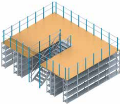
Installation de rayonnages sur 1 étage avec plateforme
