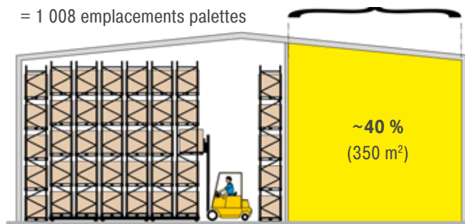
Rayonnage à palettes mobile PROmobile
